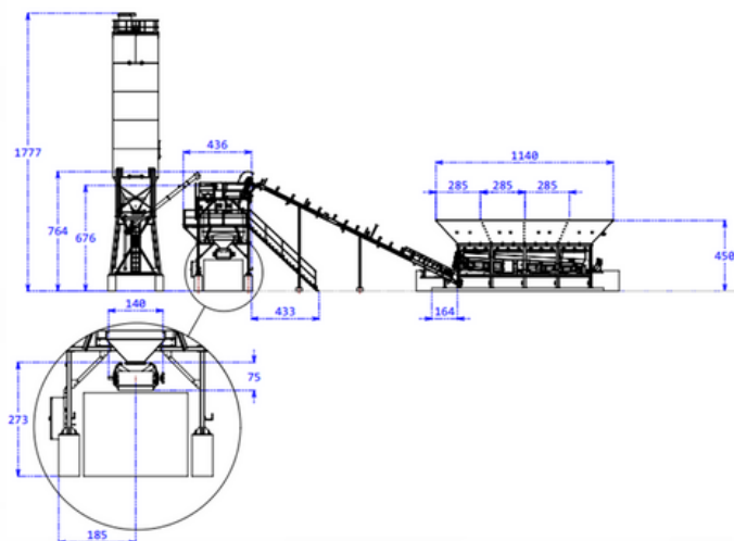
Vista lateral
